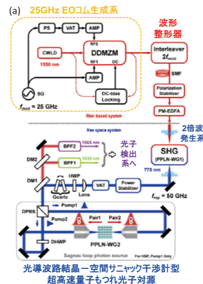
図1 a) 超高速量子もつれ光子対源の構成。電気光学変調（EOM）により高速パルス波を生成し、その二倍波を導波路型非線形光学結晶へ入射することで、量子もつれ光子対を生成する。b) 量子もつれ光子対の検出レートと励起パワーの関係。c) 量子もつれ光子対の質と励起パワーの関係。
