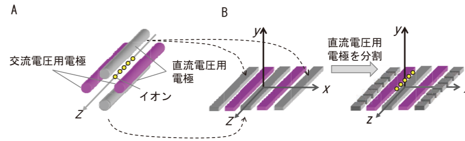
図2 イオントラップの電極構成 (A)従来型イオントラップ（リニアトラップ）、(B)オンチップイオントラップ
