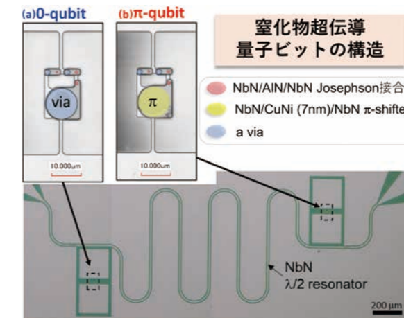
図 (a) π接合を含まない窒化物磁束量子ビット (0-qubit) と (b) π位相シフターを含む窒化物磁束量子ビット (π-qubit) と結合したNbNのλ/2コプレーナ導波路共振器の写真
