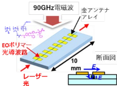
② 90GHz電磁波による直接光変調の実証
