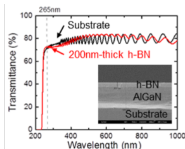
深紫外領域での高透過率（ \sim 99\% @ \lambda=265\text{nm} ）を実証
