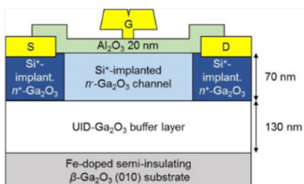
③横型微細ゲート酸化ガリウムトランジスタの開発 最大発振周波数27GHz（世界最高値）を達成
