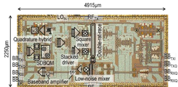
300GHzシリコンCMOSトランシーバ集積回路の顕微鏡写真
