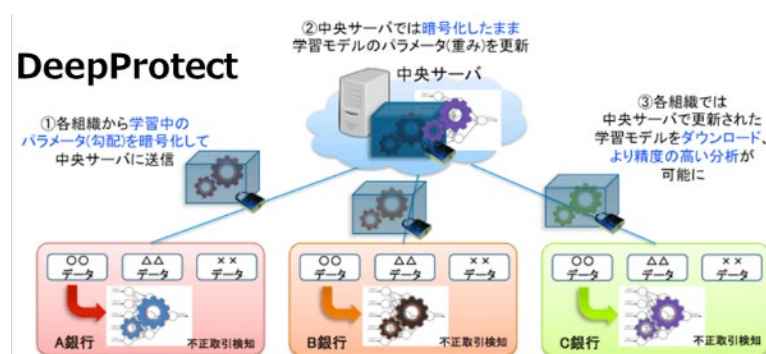
③暗号化された情報のまま機械学習を行うための秘匿協調学習技術DeepProtect
