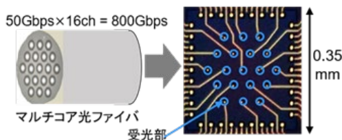
④二次元受光アレイ素子 マルチコア光ファイバと直接接続し世界初800Gbpsを達成
