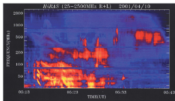
図6 2001年4月10日のフレアに伴う電波バースト
