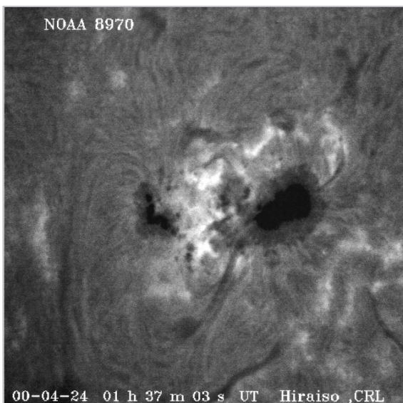
図3 H \alpha 線でみた黒点群近傍の微細構造
