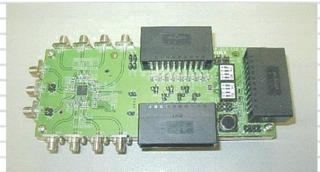
新規開発のMMICを使用したUWB送受信モジュール (インパルス方式)
