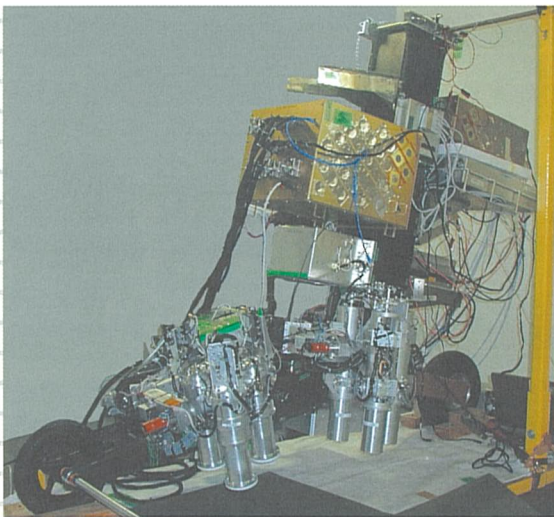
ソーラーブレン・ヘリオスの脚部に装着された47GHz帯機械駆 動型マルチビームホーンアンテナシステム及びIP伝送用中継器
