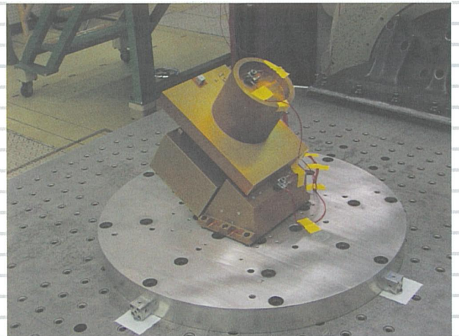
WCI(広視野コロナ撮像装置)の熱 構造モデルを用いた振動試験風景
