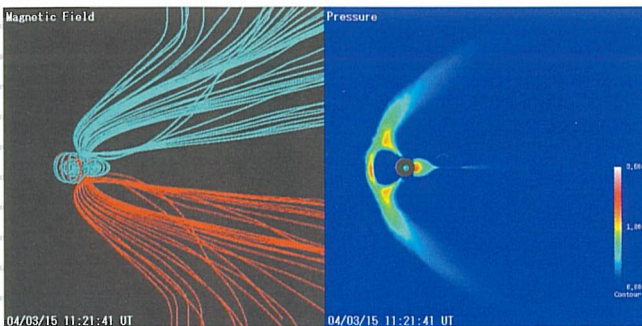
スーパーコンピュータを用いた 「宇宙天気予報」の公開図の一部
