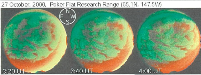
アラスカにおいてCRLの装置で初めて発見された、 形が変わらないオーロラ
