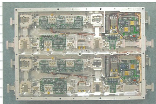
開発された送受信機部BBM (四つの T/Rユニットを含む)の外観と内部
