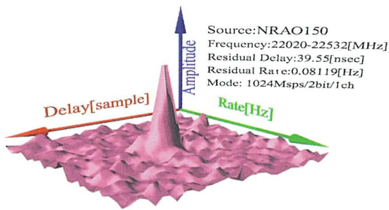
日-フィンランドe-VLBI実験の2Gbps観測で得られたフリッジ
