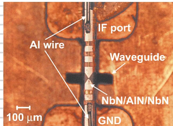
90GHz帯導波管型NbN SISミキサ
