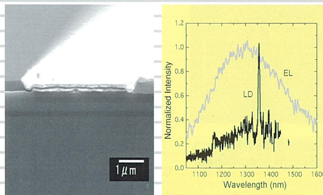
作製した量子ドットレーザの側面図と波長1.3 μmでの発振スペクトル
