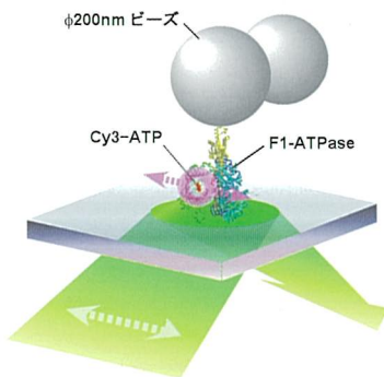
偏光検出型TIRF (全反射蛍光励起システム) の概念図
