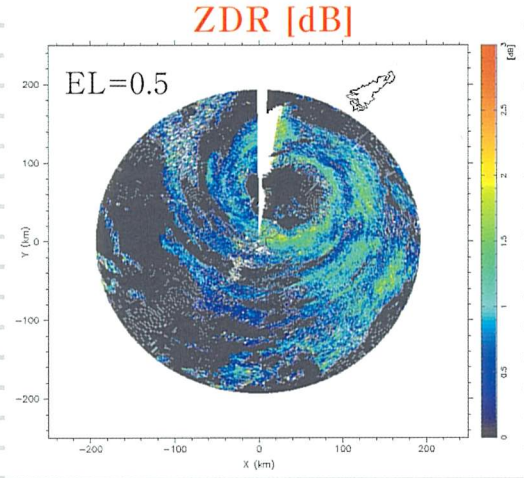
降雨レーダで観測した台風10号(平成15年8月7日) (水平面分布)
