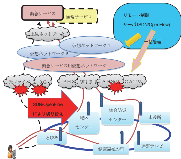
図2 岩手県遠野市における SDN を用いた有無線統合 NW 制御に関する実証
