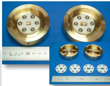
(b) 縦型Ga 2 O 3 デバイスの高耐圧化の研究開発用試料台の設計・試作 (未来ICT研究所)
