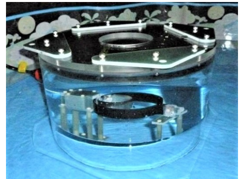
(c) 海中電波伝搬実験 (アンテナ部) (ワイヤレスネットワーク総合研究センター)
