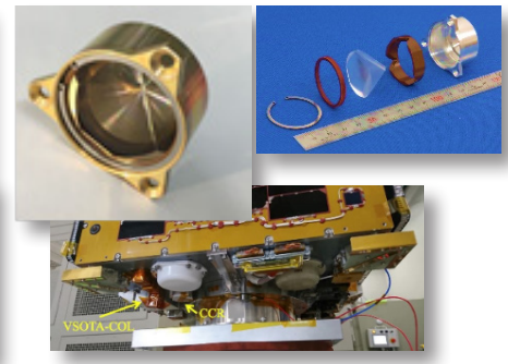
(c) RISESAT (平成31年1月に打ち上げ成功) 搭載の超小型光送信機のコーナーキューブリフレクターのホルダーを設計・製作 (ワイヤレスネットワーク総合研究センター)
