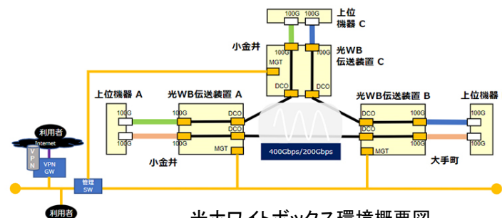
光ホワイトボックス環境概要図
