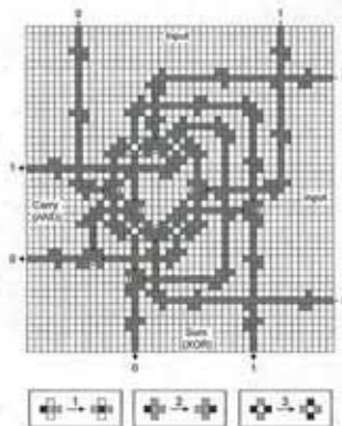
図1 半加算器のブラウンセルオートマトンにおける局所形状 (1) (2) (3) の選移ルールによって2つのビットが加算される。加算の動作が計算の基本になる。
