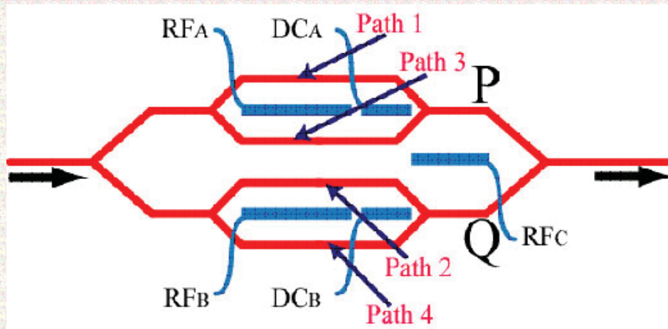
図1: 光FSK変調器の構造。2つのマッハツェンダー構造からなる。RFA, RFBに90度の位相差をもつ正弦波信号を入力する。この信号の周波数がFSKの周波数変位量に一致する。また、RFCの電圧で光周波数の切り替えが可能である。ラベル信号をRFCに供給することでラベル情報をFSK信号に変換することができる。
