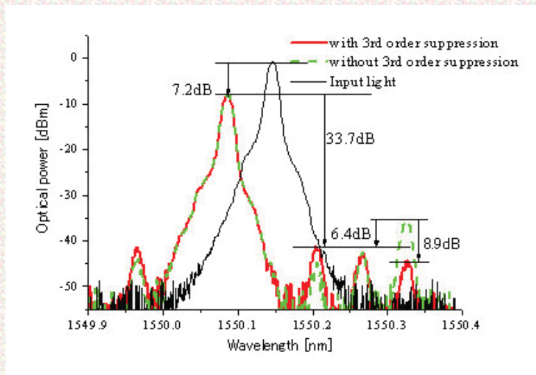
図2: 光FSK変調器による光周波数シフトの一例。黒線は入力光スペクトル。緑線と赤線は出力光スペクトル。波長(光周波数)がシフトした成分が生成されている。赤線は不要な成分(3次高調波)を抑圧するための補償を行ったもの。
