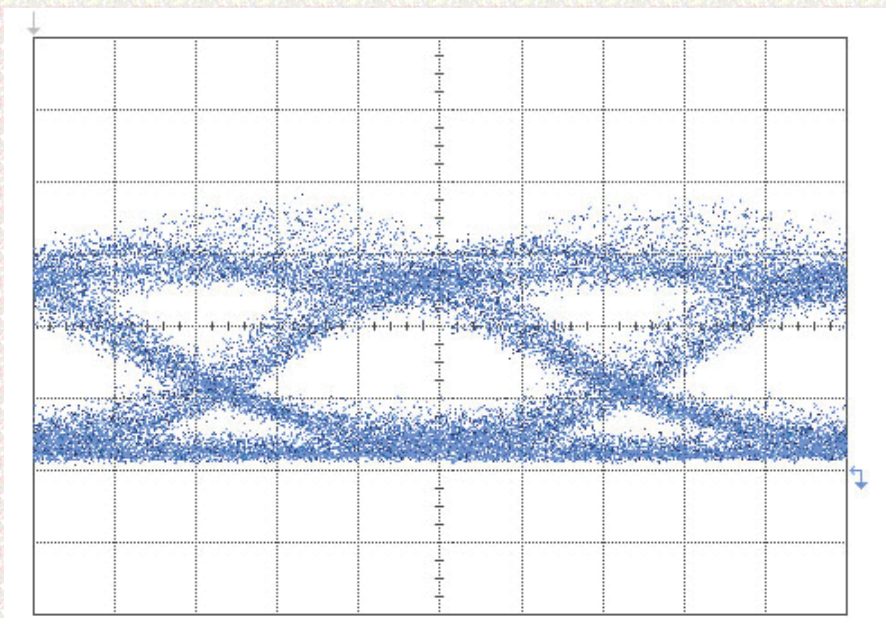
図3: 95km伝送後に復調されたFSK信号。FSK信号は光フィルタと光検出器の組み合わせで復調できる。
