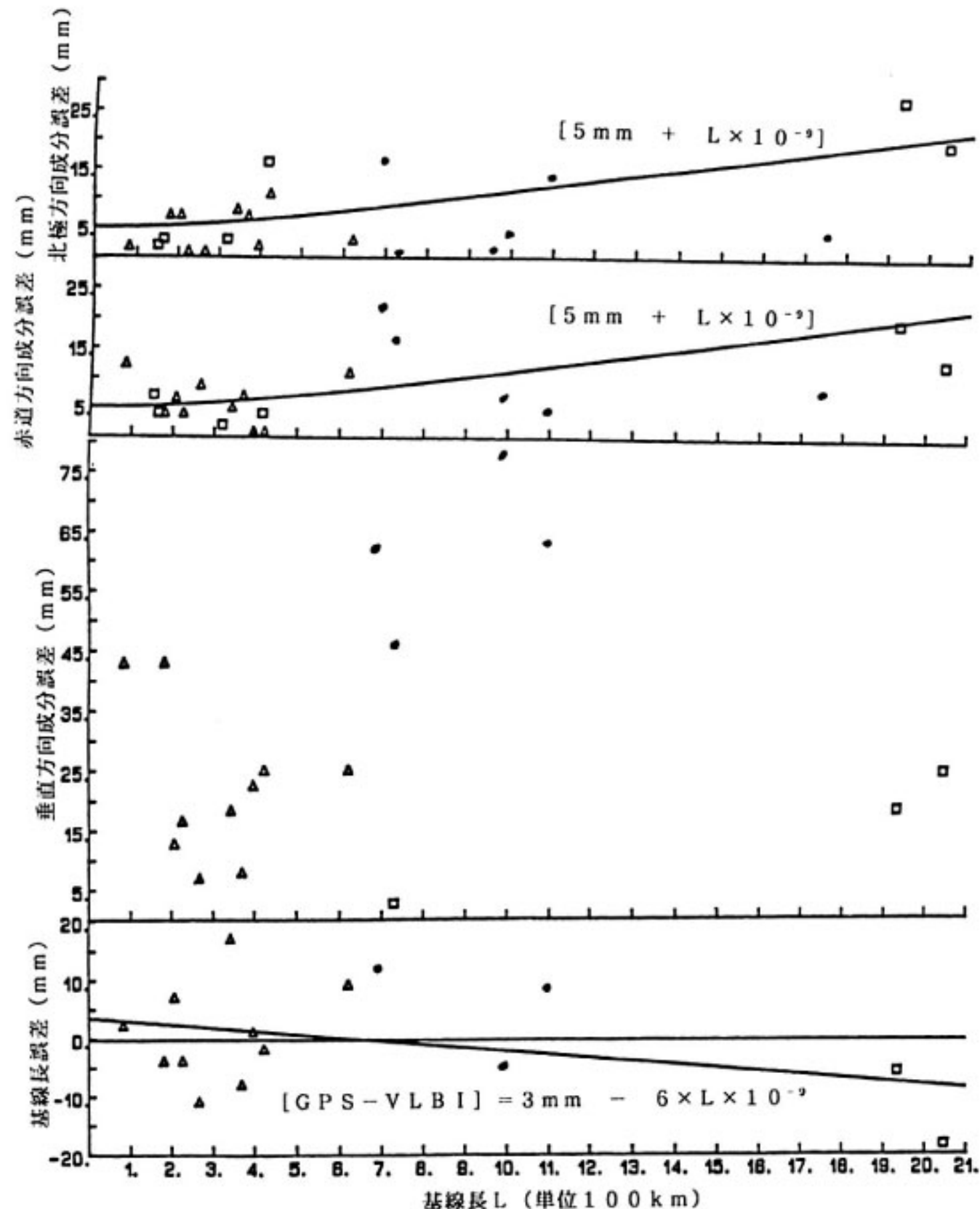
第9図 VLBI と GPS のコロケーション結果。縦軸はコロケーション誤差の各成分。横軸は基線長
