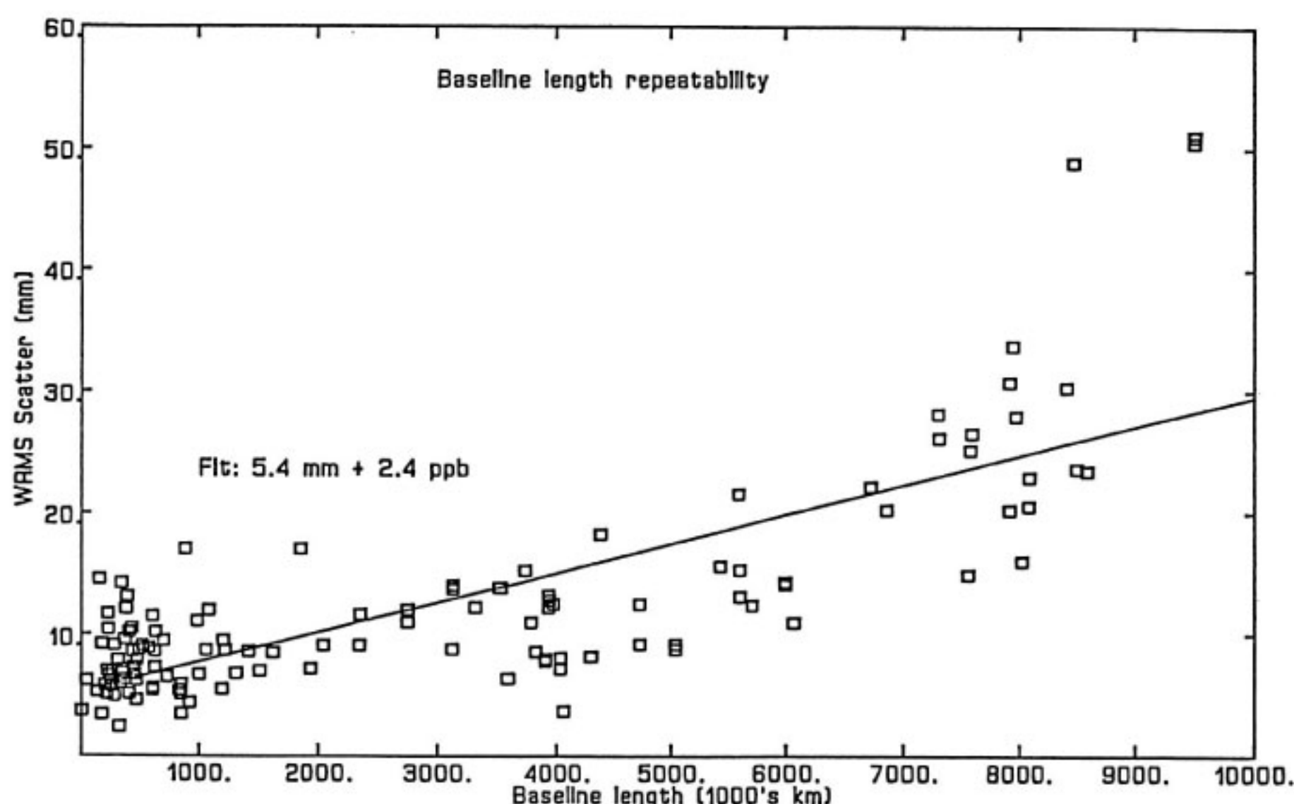
第8図 VLBI測距精度の再現性。縦軸は再現性誤差、横軸は基線長。
