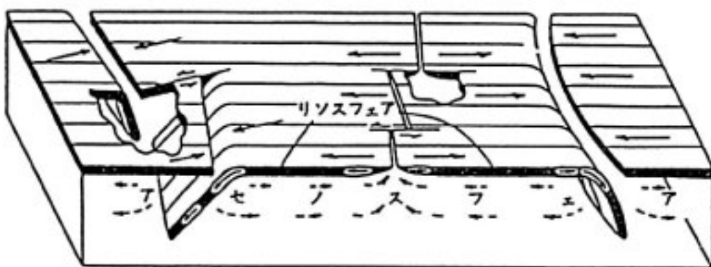
第11図 プレート運動の模式図
