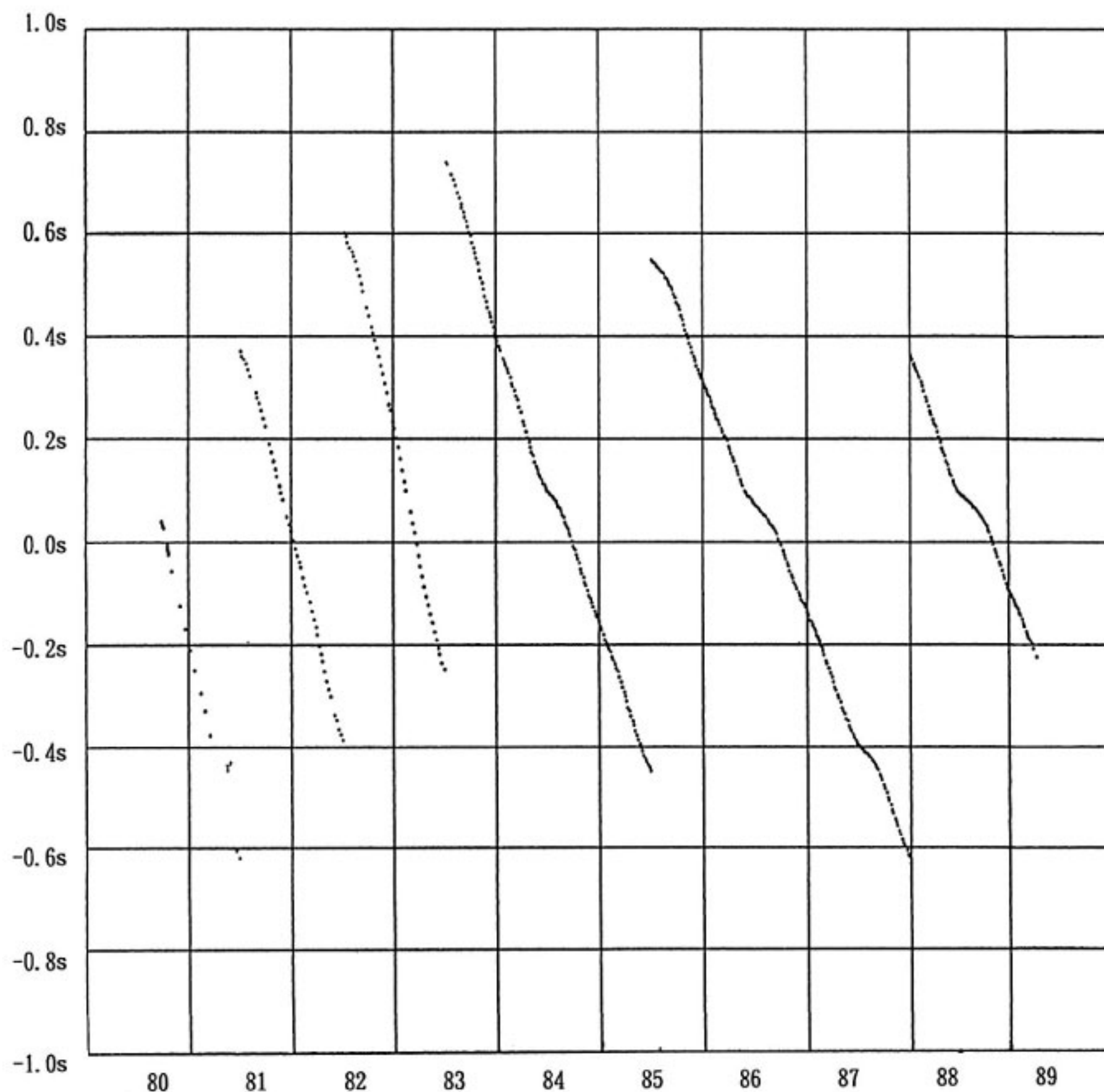
第15図 最近10年間の地球回転の変化
