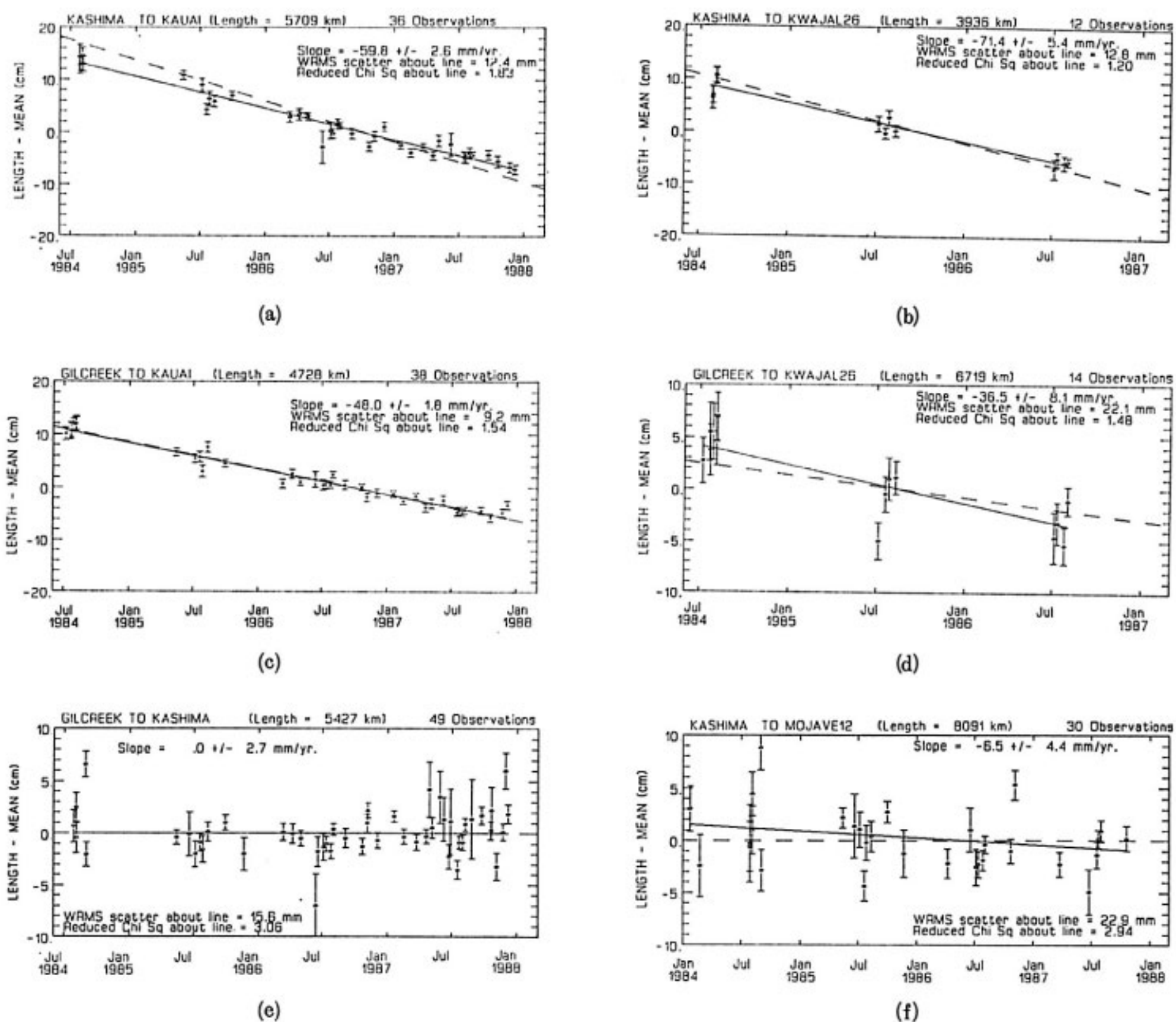
第13図 日米太平洋実験参加の各基線毎の基線長変化の測定結果
