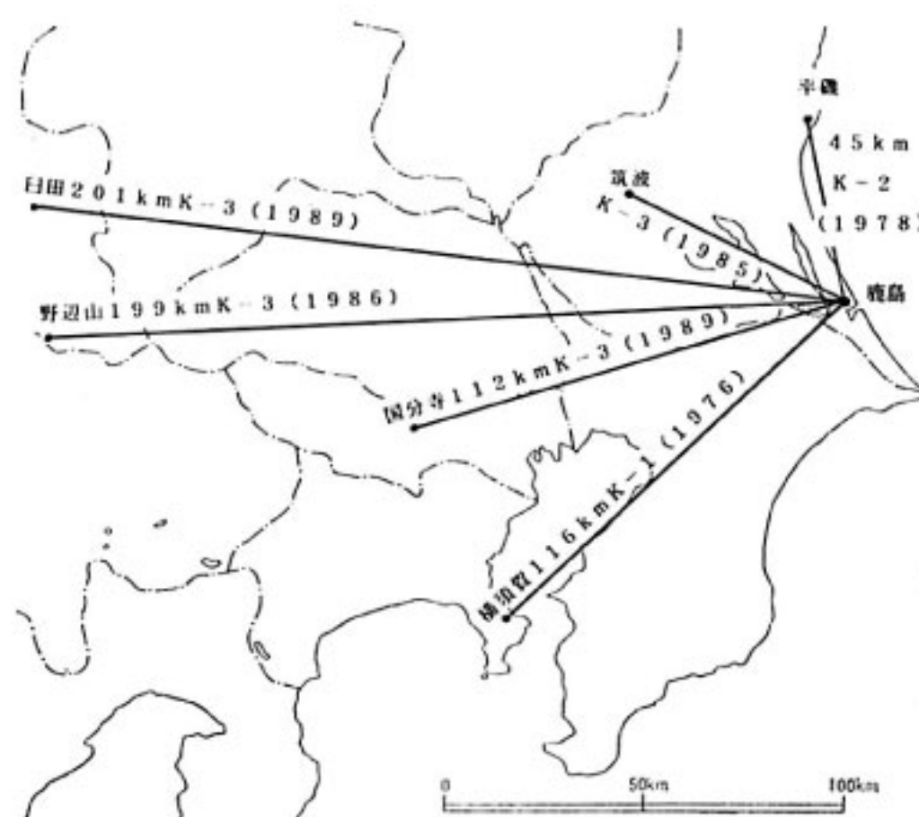
第5図 関東地方の VLBI 局の配置図
