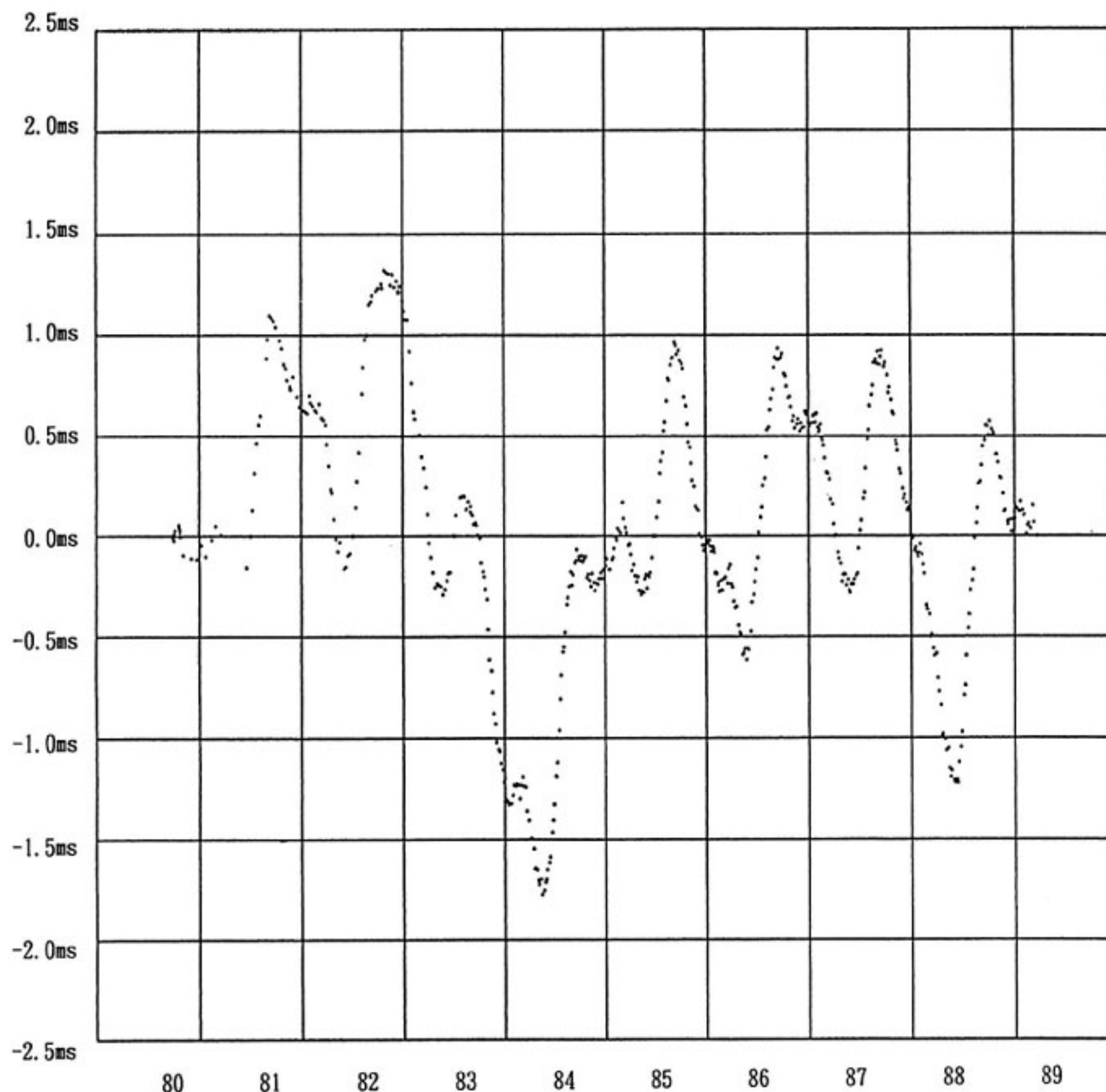
第16図 1日の長さの変化、第15図微分
