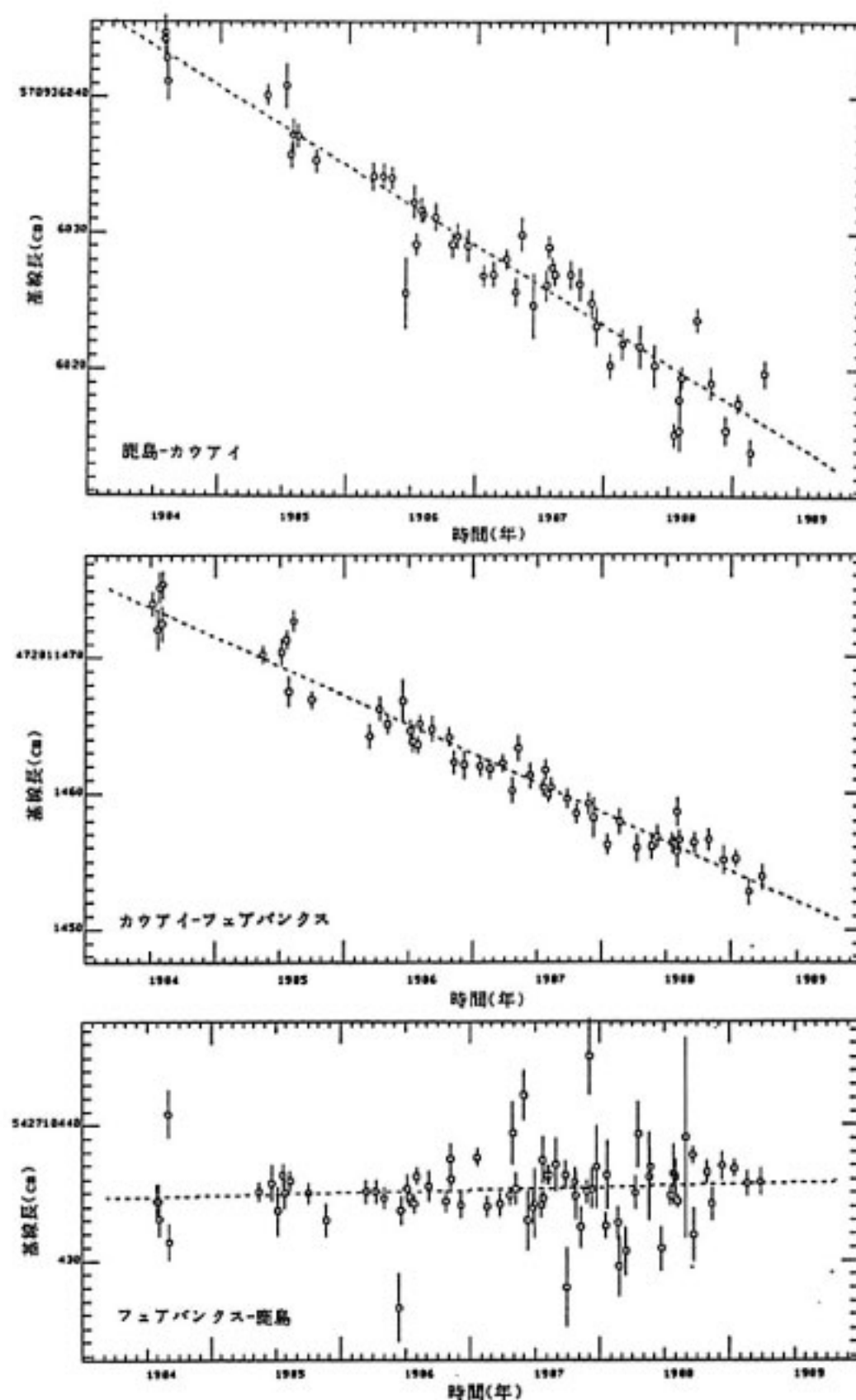
第3図 CDP 実験で得られた1984年から1989年始めまでの鹿島-カウアイ(ハワイ)、カウアイ-フェアバンクス(アラスカ)、フェアバンクス-鹿島の基線長変化。横軸は時間(一目盛り一ヶ月)、縦軸は基線長(一目盛り1cm)。各データは一回の実験で求められた基線長と正規誤差を示す。破線は重み付き最小自乗法で求めた直線で、その傾きは上から -5.9 \pm 0.2 cm/年、 -4.3 \pm 0.1 cm/年、 0.2 \pm 0.2 cm/年である。
