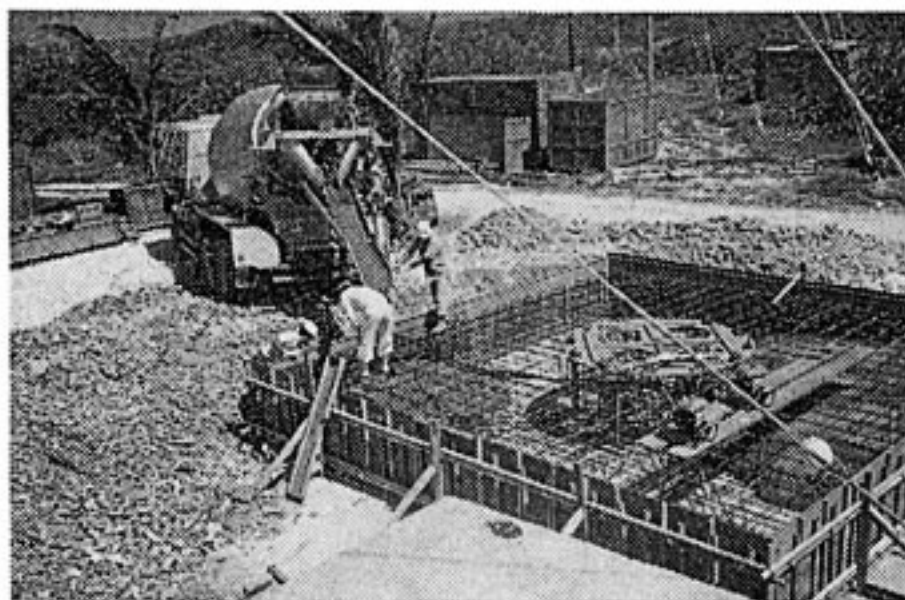
第18図 10メートルアンテナの基礎工事
