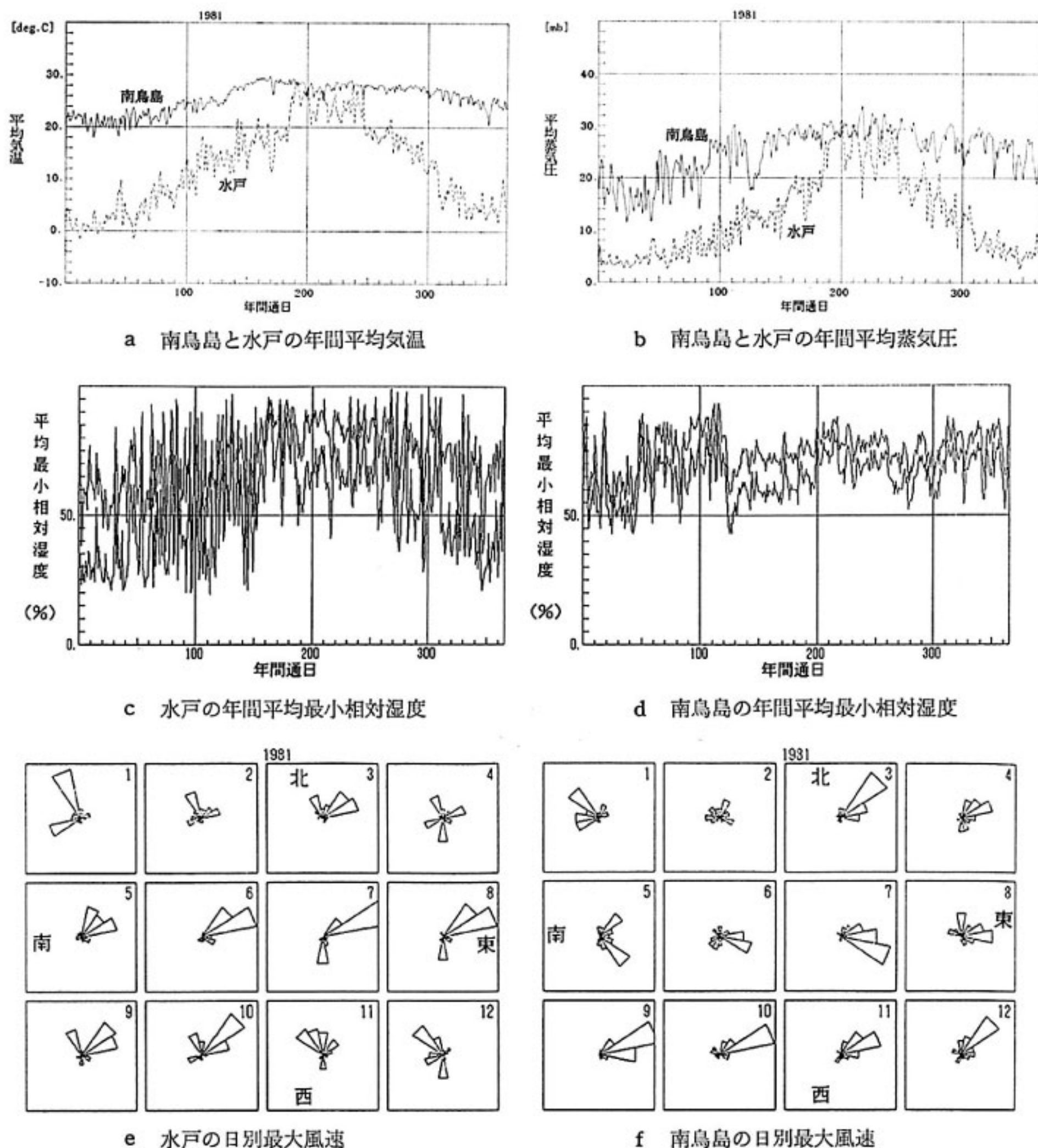
第5図 南鳥島と水戸の気象の比較
