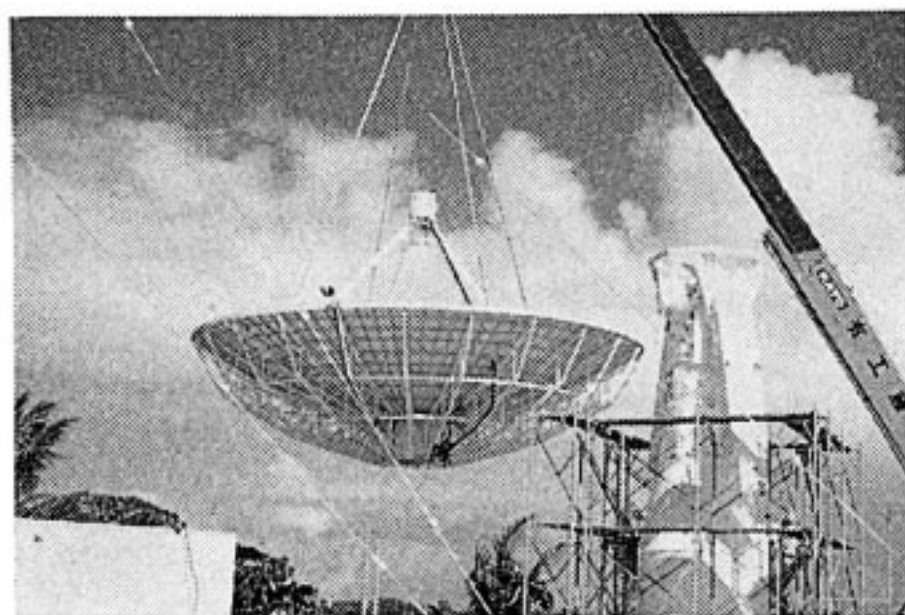
第20図 アンテナディッシュ部取り付け
