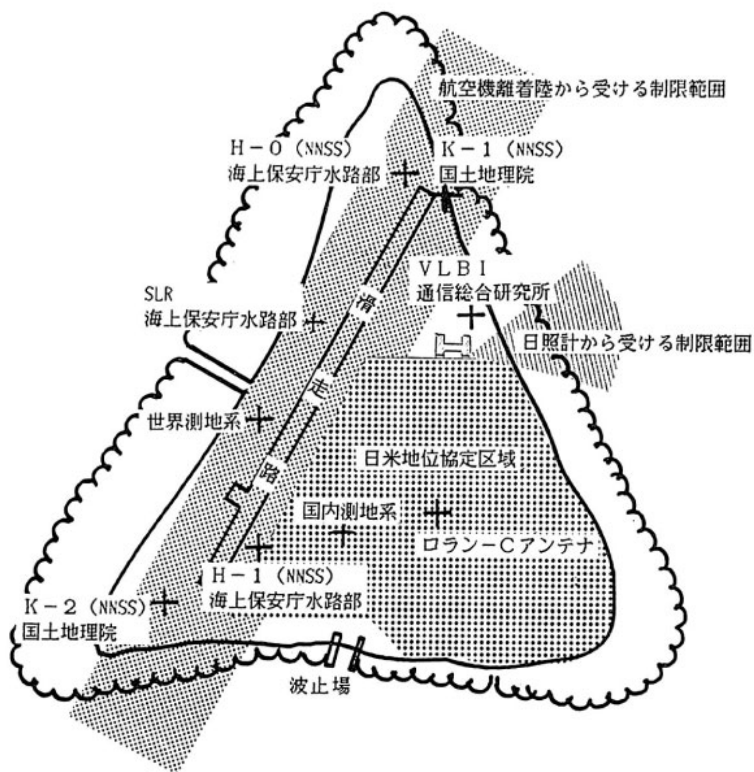
第3図 各測量点の配置およびアンテナ建設可能範囲
