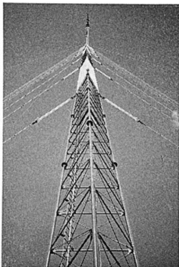
第11図 ロラン-Cのアンテナ 高さ110メートルのトッ プローディングアンテナ
