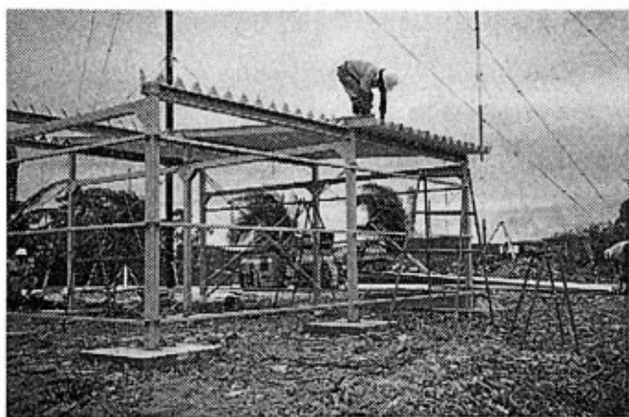
第15図 資材収納用倉庫 NO 組み立
