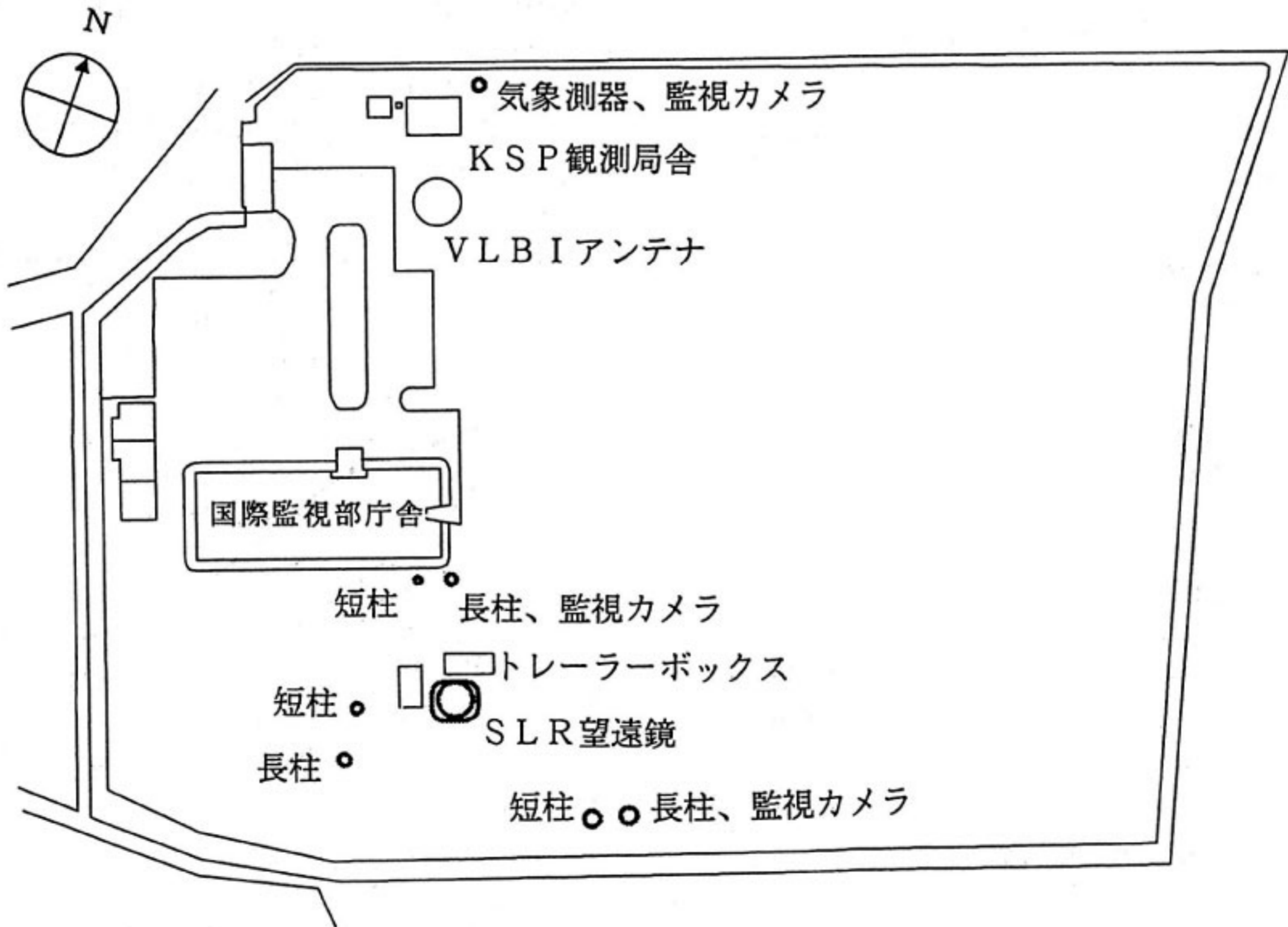
第4図 国際監視部内 KSP 観測施設配置
