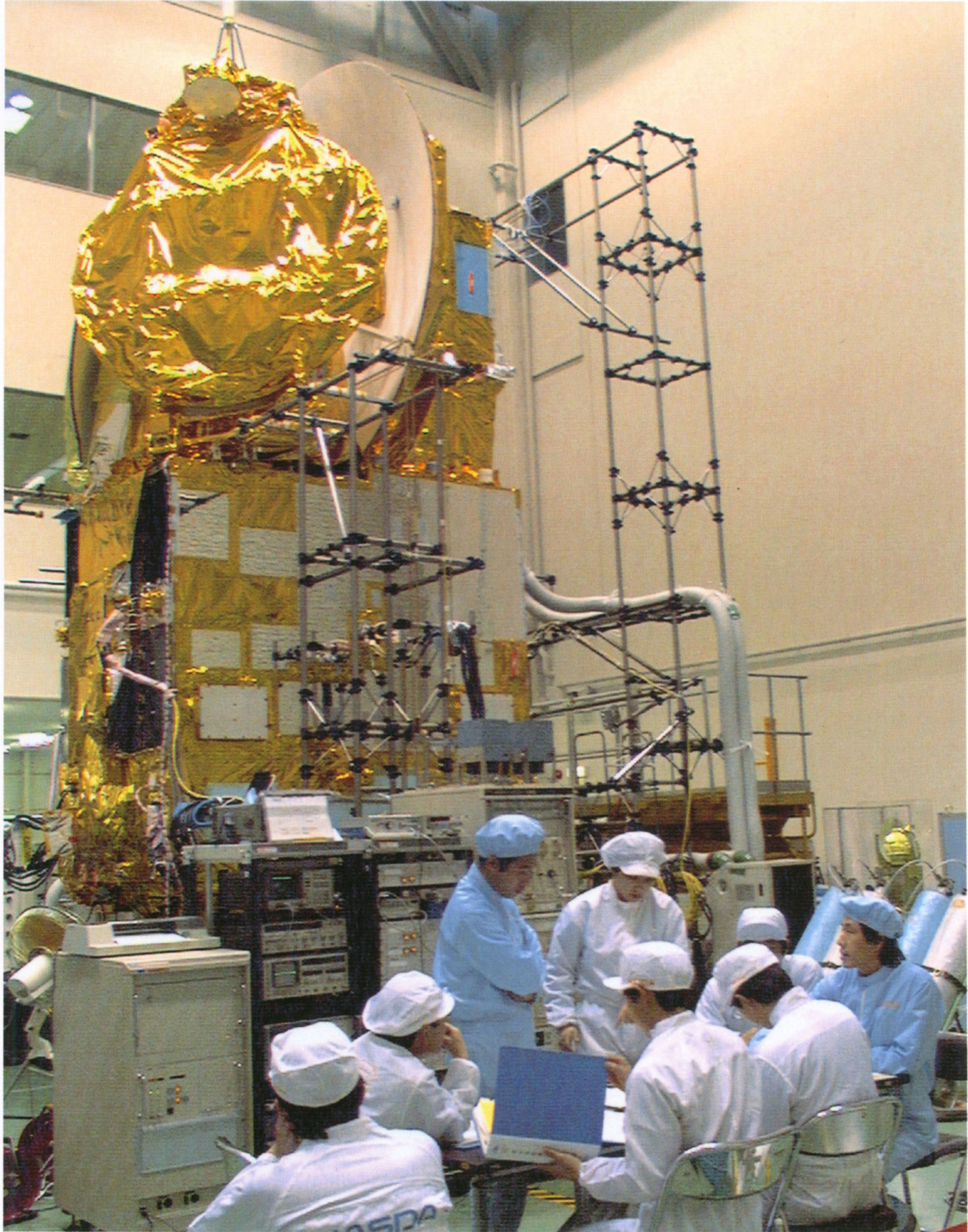
COMETS 打ち上げ前試験風景
