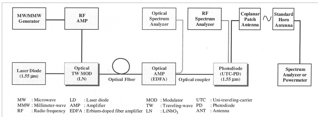
図1 光変調、フォトディテクション、光給電アンテナ及び放射・受信実験系
