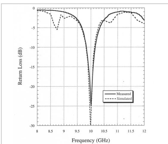
図 6 CPA の反射特性
