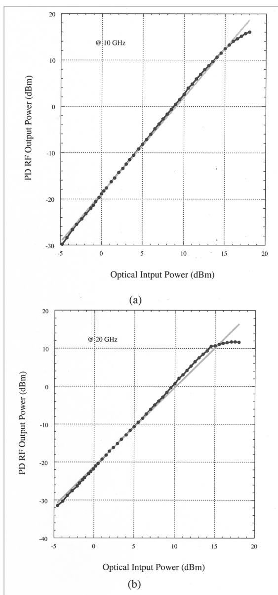
図3 フォトディテクターからのRF出力 (a) 10GHzと(b) 20GHz
