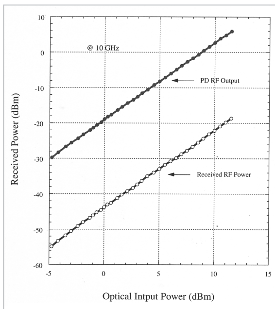
図9 PDへの光入力に対するRF出力及び受信アンテナでのパワーレベル
