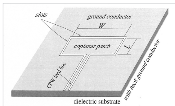
図4 共平面給電構造を有する共平面パッチアンテナ (CPA)
