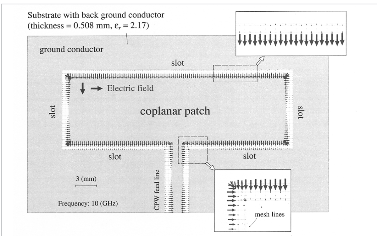
図 5 共平面パッチアンテナにおける電界分布
