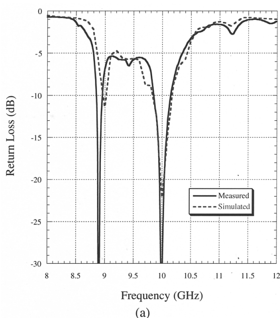
図8 CPAの(a)反射特性と(b)放射パターン
