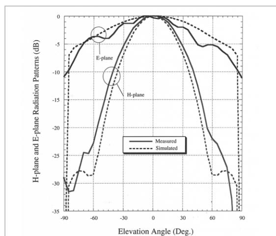
図 7 放射パターン
