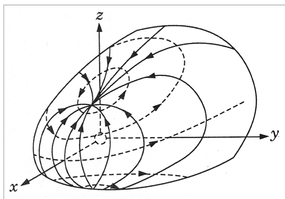
図2 磁気圏境界面の3次元表示。実線は磁力線を、点線は境界面を流れる電流を示す(Midgely, 1963)
