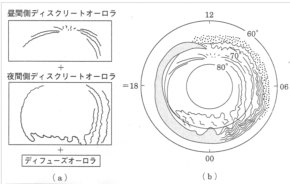
図8 オーロラオーバルを構成するディスクリートオーロラと、ディフューズオーロラ。磁力線に沿って上向きの電流が流れる領域で、ディスクリートオーロラは激しく輝く
