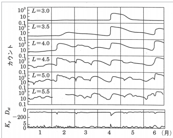
図 13 1 MeV 以上の放射線電子に対する磁気嵐の影響。地球からの距離を変えて、それぞれの場所でのフラックスの時間変動を示す (Walt, 1994)
